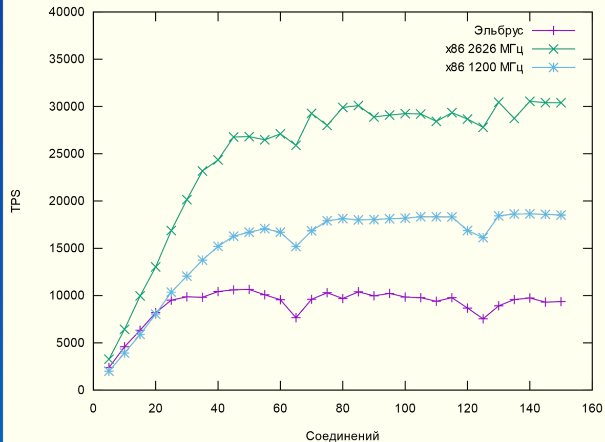
TPC-B транзакций в сек
