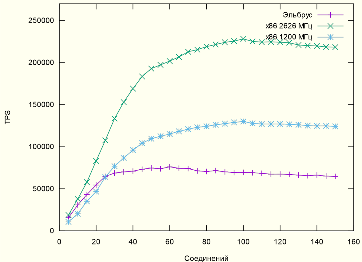
SELECT транзакций в сек
